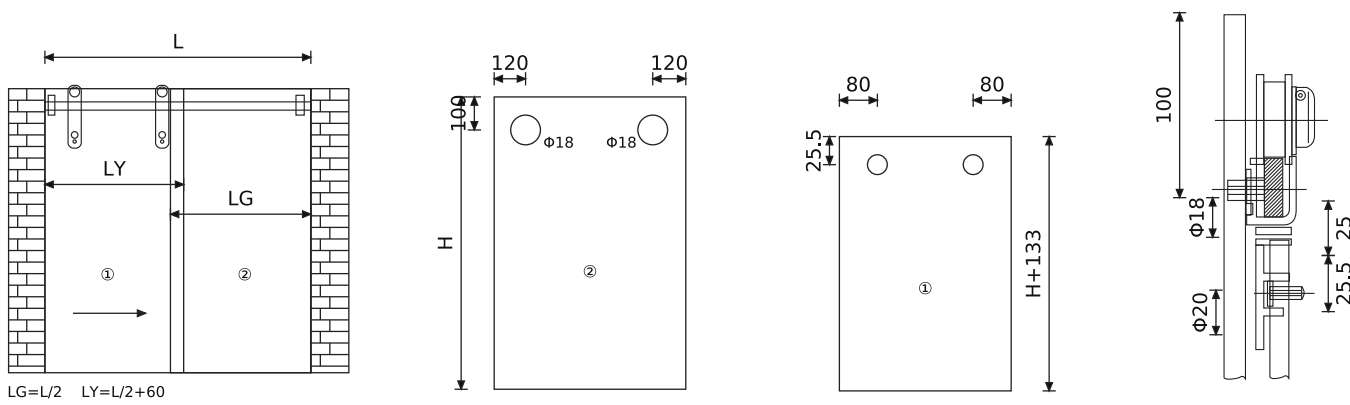
30X10 方管平面安装图 Installation map with 30X10 Square pipe
